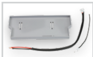
Instalační kit E 124 pro záložní zdroj bez baterií. Standardní baterie 12V/4Ah
