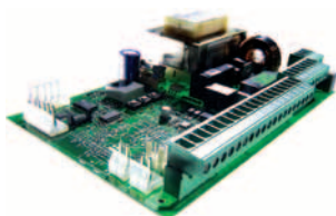
řídící jednotka JE275 pro sloupy může ovládat až 4 sloupy
