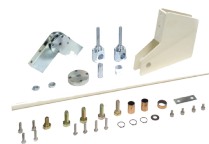
Kloubový kit pro zlamo- vací obdélníková ráhna (max. výška stropu 3 m)
